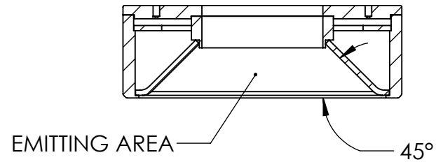
SECTION A-A SCALE 1 : 2
