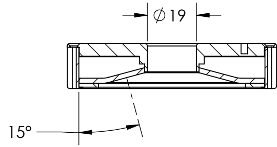
SECTION A-A SCALE 1 : 1.5
